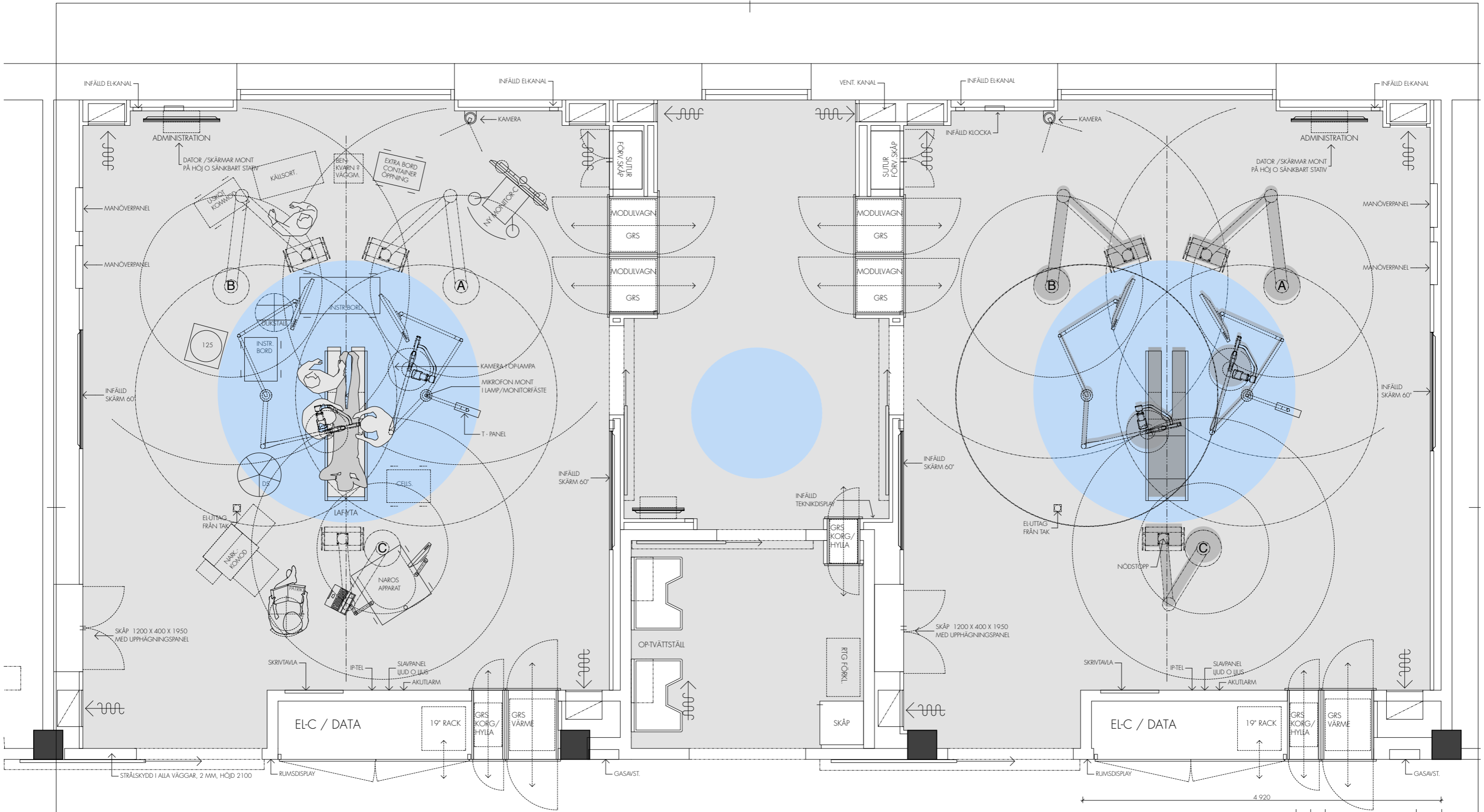
OPERATIONSSAL, VÄNSTER, 59.4 m 2
